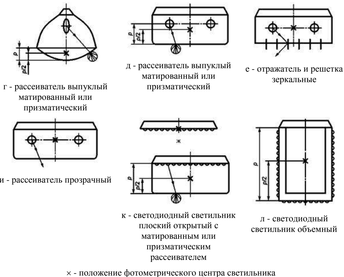
Рисунок В.1 - Положение фотометрического центра осветительного прибора
