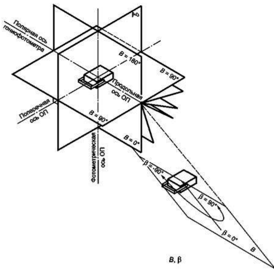
Рисунок Б.1 - Системы фотометрирования, лист 1
