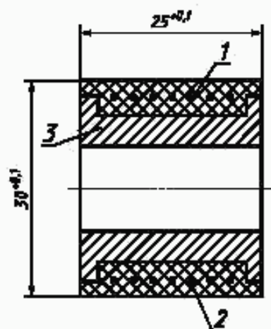
1 — покрытие из токопроводящей резины; 2 — проводящий бандаж; 3 — латунная втулка
