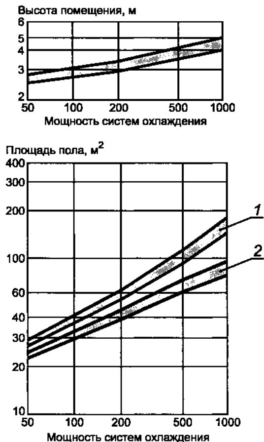
Рисунок А.6 - Высота и площадь пола зон с холодильными установками и системами подготовки воды
