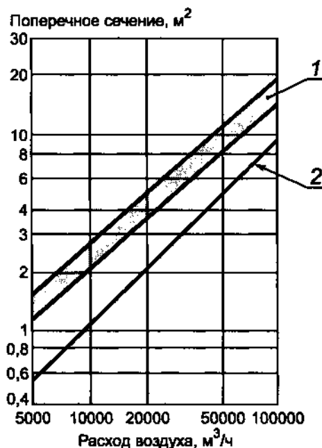
Рисунок А.7 - Поперечное сечение шахт
