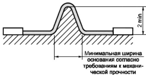
Рисунок Е.1 - Размеры ребер
