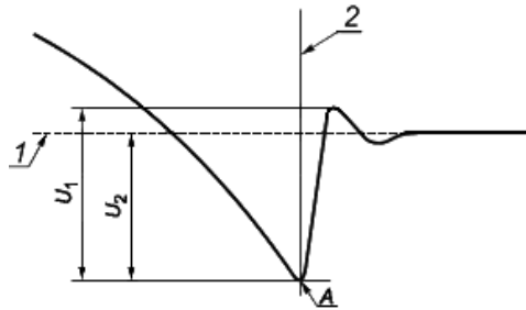
Рисунок С.1 - Определение фактического значения коэффициента \gamma
