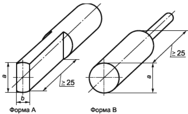
Рисунок 5 - Щупы (см. 9.2.4.5)
