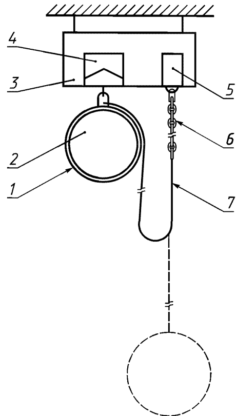
1 — пояс; 2 — груз или манекен массой 100 кг; 3 — подъемное устройство; 4 — распепляющее устройство; 5 — датчик измерительного устройства; 6 — технологический фал для удлинения стропа до 2 м или до двух длин стропа; 7 — строп
